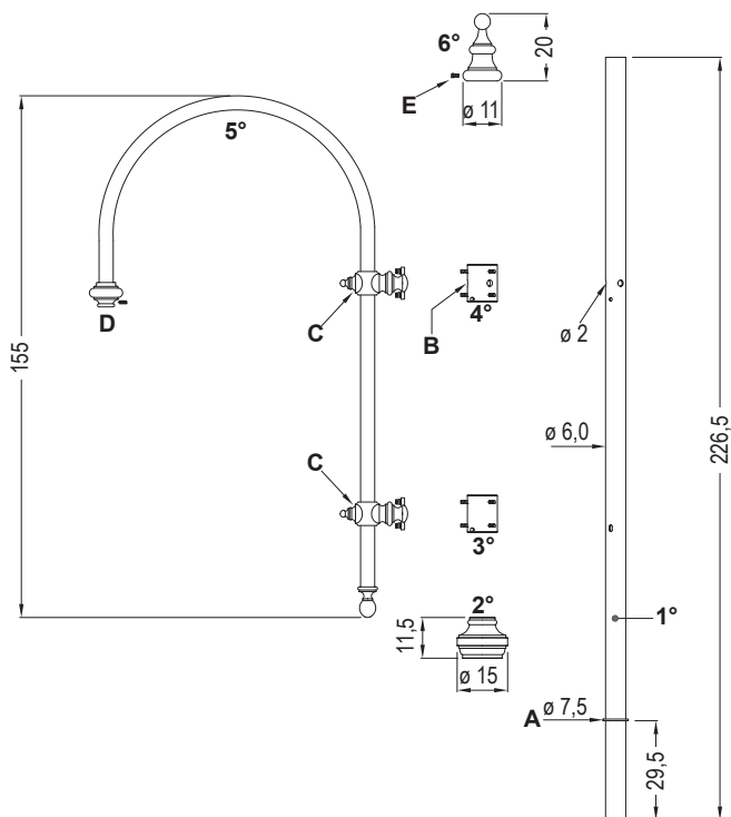
Esploso
