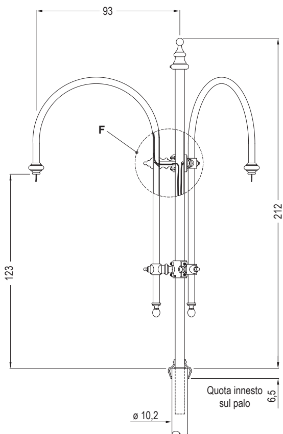
Sezione - Prospetto
