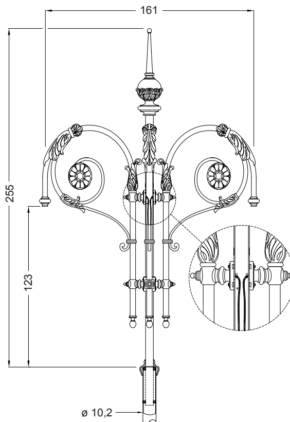
Prospetto - Sezione particolare
