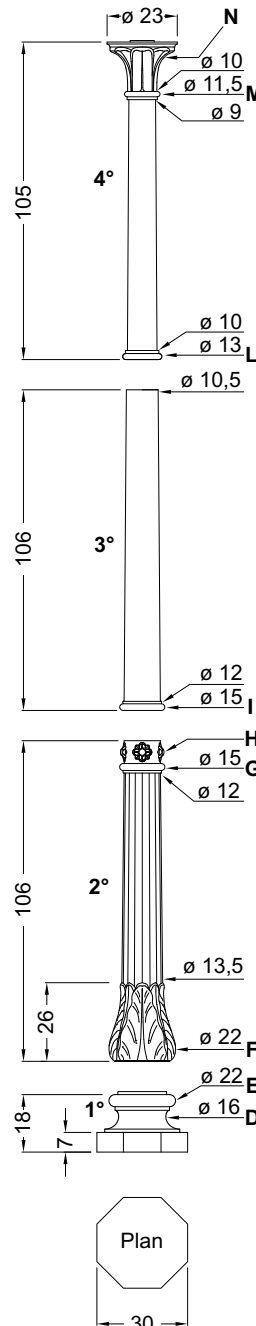
Éclaté
