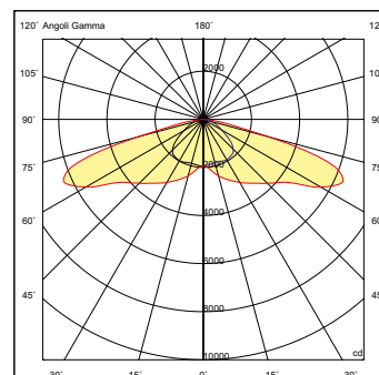
Type I (NLG 19) Stradale - Posizione centro strada
