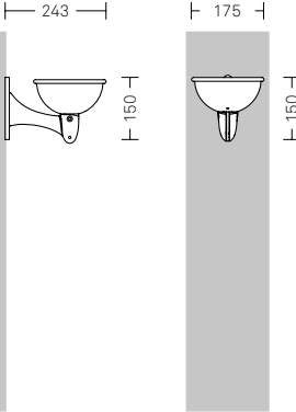
Melia – a parete 2800.000 Posacenere oscillante per svuotare la cenere • Ghisa
