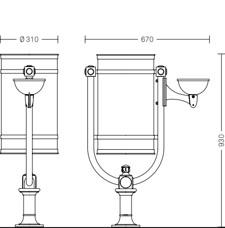
Melia 2274.002 M • Ghisa e acciaio zincato • Capacità 37l
