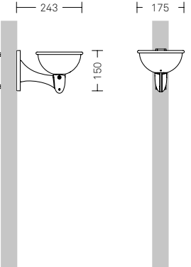
Melia – per tubi 2800.001 V 2800.002 V 2800.003 V Posacenere con placca per tubi da: Ø 33mm (2800.001) Ø 48mm (2800.002) Ø 60mm (2800.003) • Ghisa
