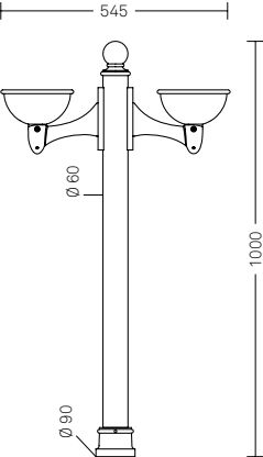
Melia – a colonna 2800.005 M • Ghisa e acciaio zincato
