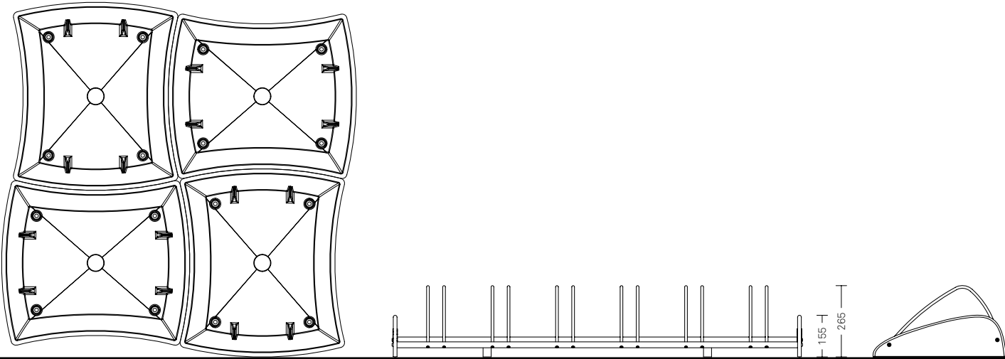
Portabici 2285.000 T 6 posti • Ghisa e acciaio zincato
