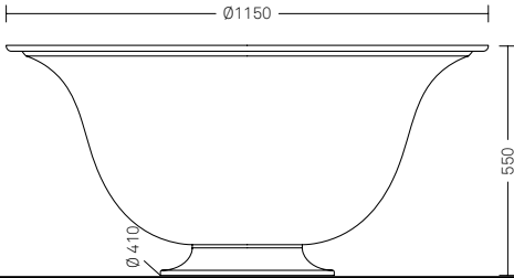
Salix 2204.000 T • Ghisa • Capacità 200l
