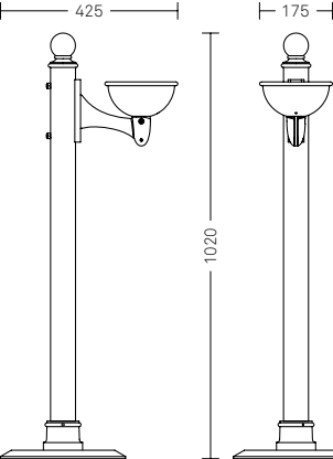
Melia – a piantana 2800.004.001 P • Ghisa e acciaio zincato
