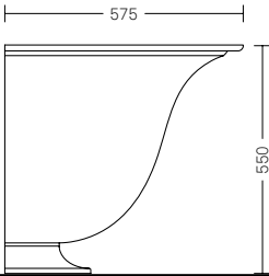
Salix – a parete 2204.001 T • Ghisa • Capacità 100l
