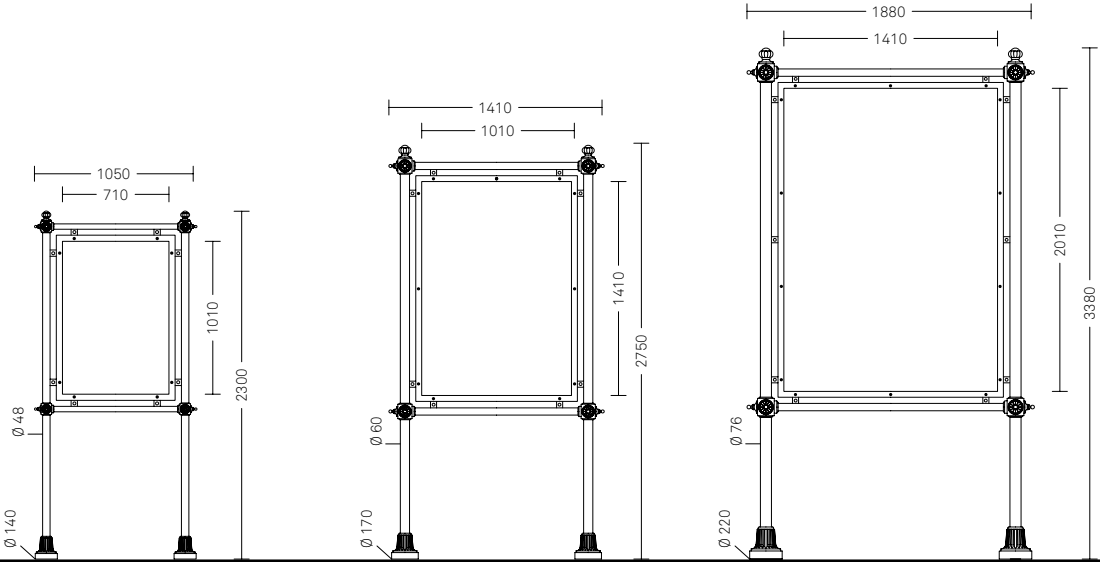
Stendardo verticale 2291.000.500 M
