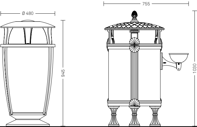
Idesia 2277.002 T • Alluminio e acciaio zincato • Capacità 75l
