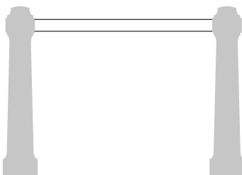
Tubo 9522.842 Accessorio per transenna al metro lineare • Acciaio zincato a caldo e verniciato • Ø 42mm x 3mm di spessore
