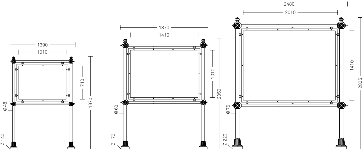
Stendardo orizzontale 2291.000.600 M
