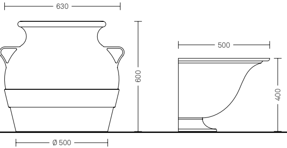
Layia 2212.000.001 T • Ghisa • Capacità 125l
